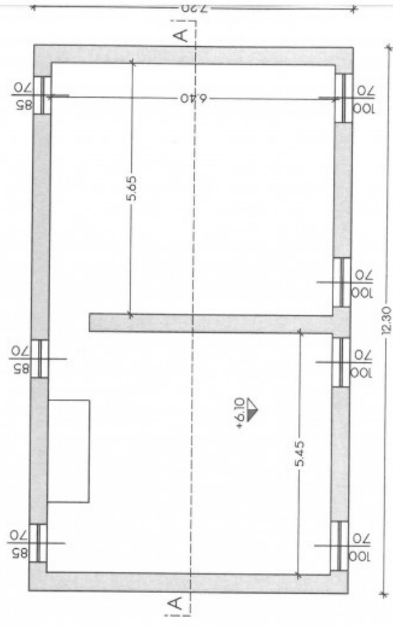
PIANTA SOTTOTETTO
